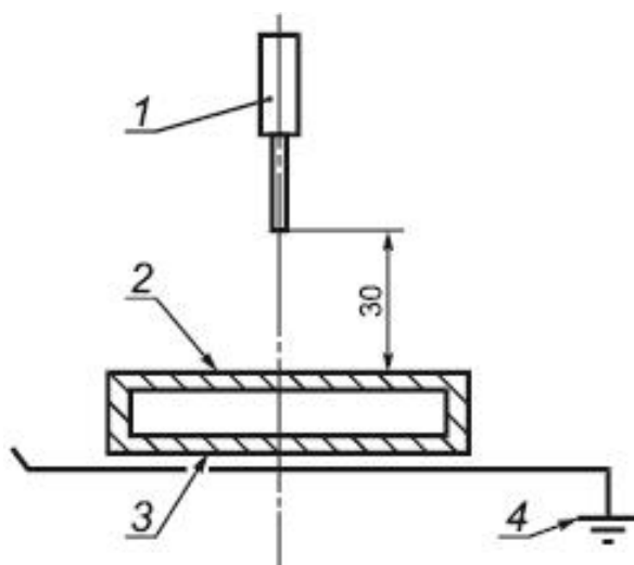
Рисунок 8 - Электризация корпуса в электрическом поле источника высокого напряжения постоянного тока
