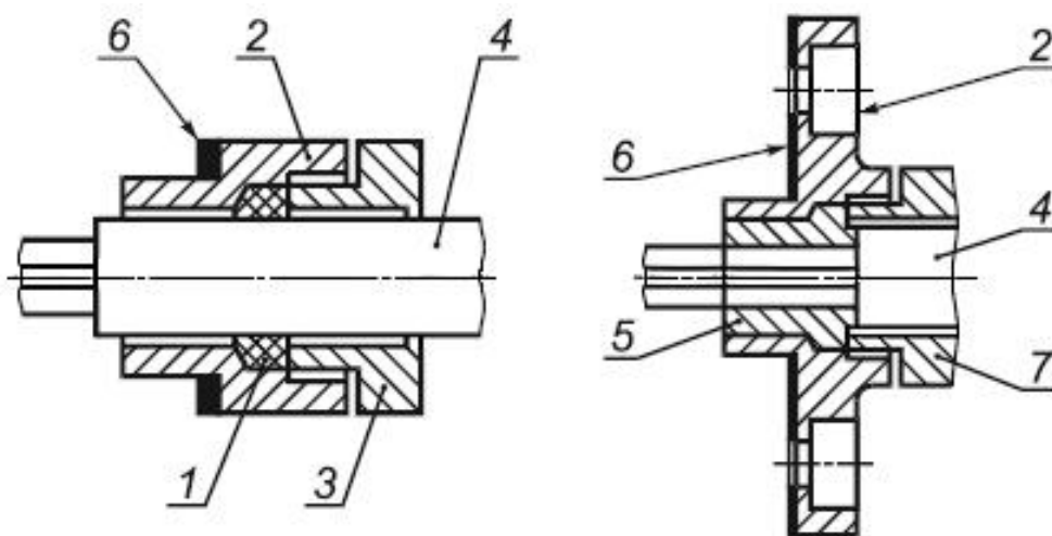
Рисунок А.1 - Кабельные вводы
