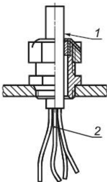
а) Кабельный ввод
