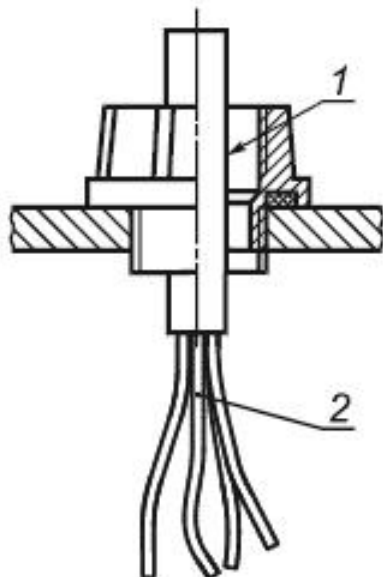
b) Трубный ввод
