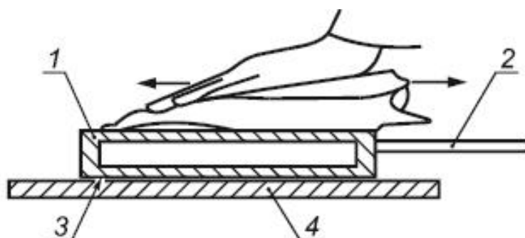
Рисунок 6 - Электризация методом трения-скольжения с использованием полиамидной или хлопковой ткани
