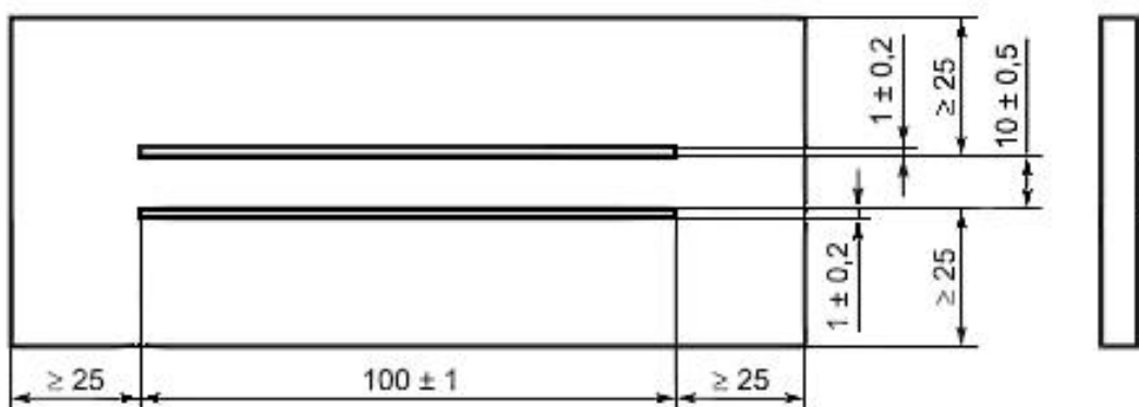
Рисунок 5 - Испытуемый образец с электродами из проводящей краски
