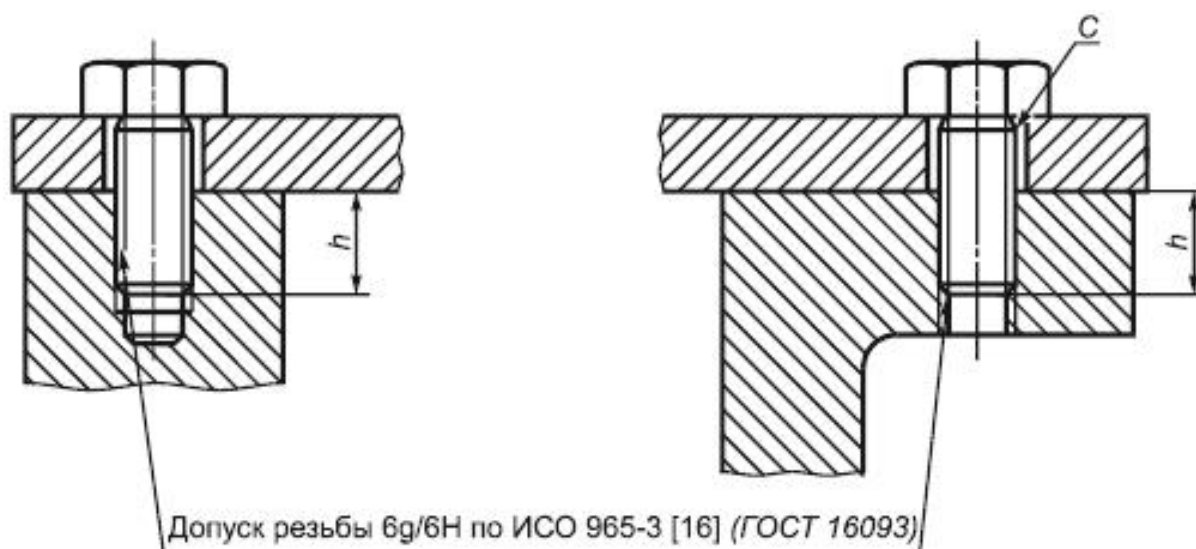
Рисунок 1 - Допуски и зазор для резьбовых крепежных деталей
