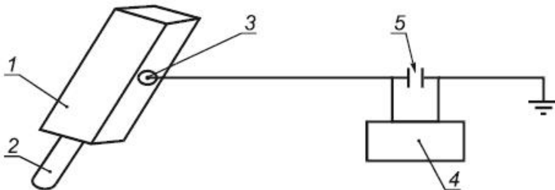
Рисунок 7 - Разряд наэлектризованного корпуса посредством зонда, заземленного через конденсатор емкостью 0,1 мкФ
