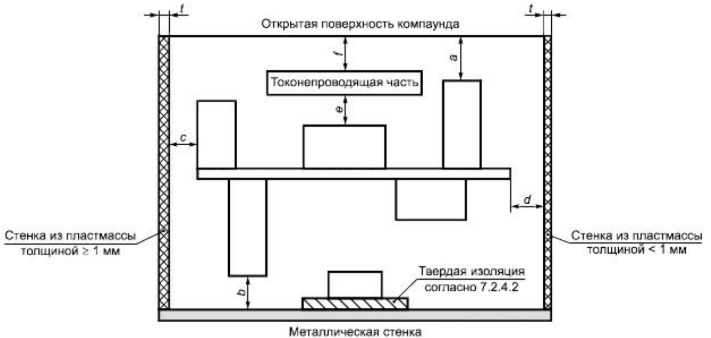
Рисунок 1 - Расстояния в компаунде
