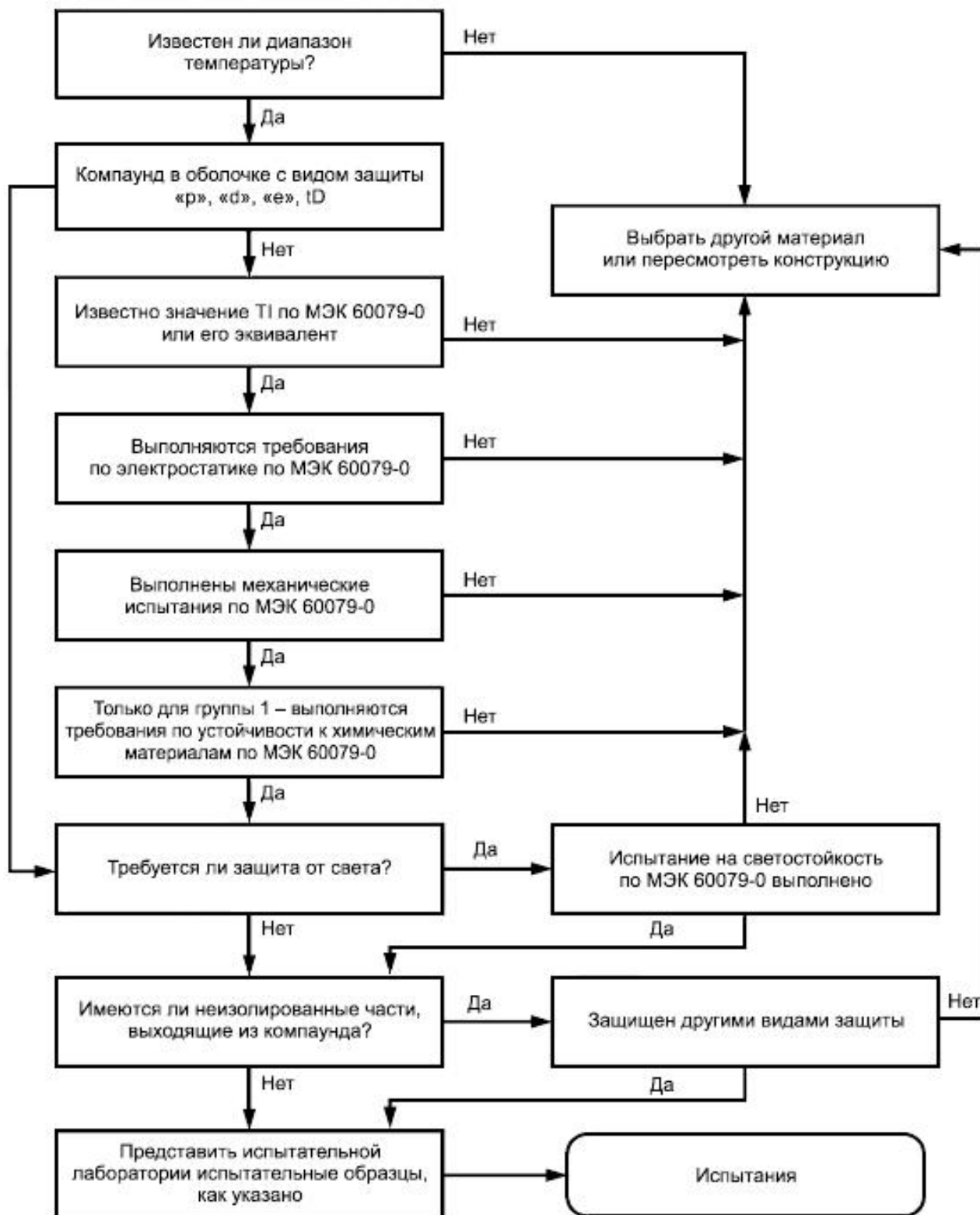
Рисунок А.1 - Основные требования к компаундам для оборудования с взрывозащитой вида "герметизация компаундом "m"
