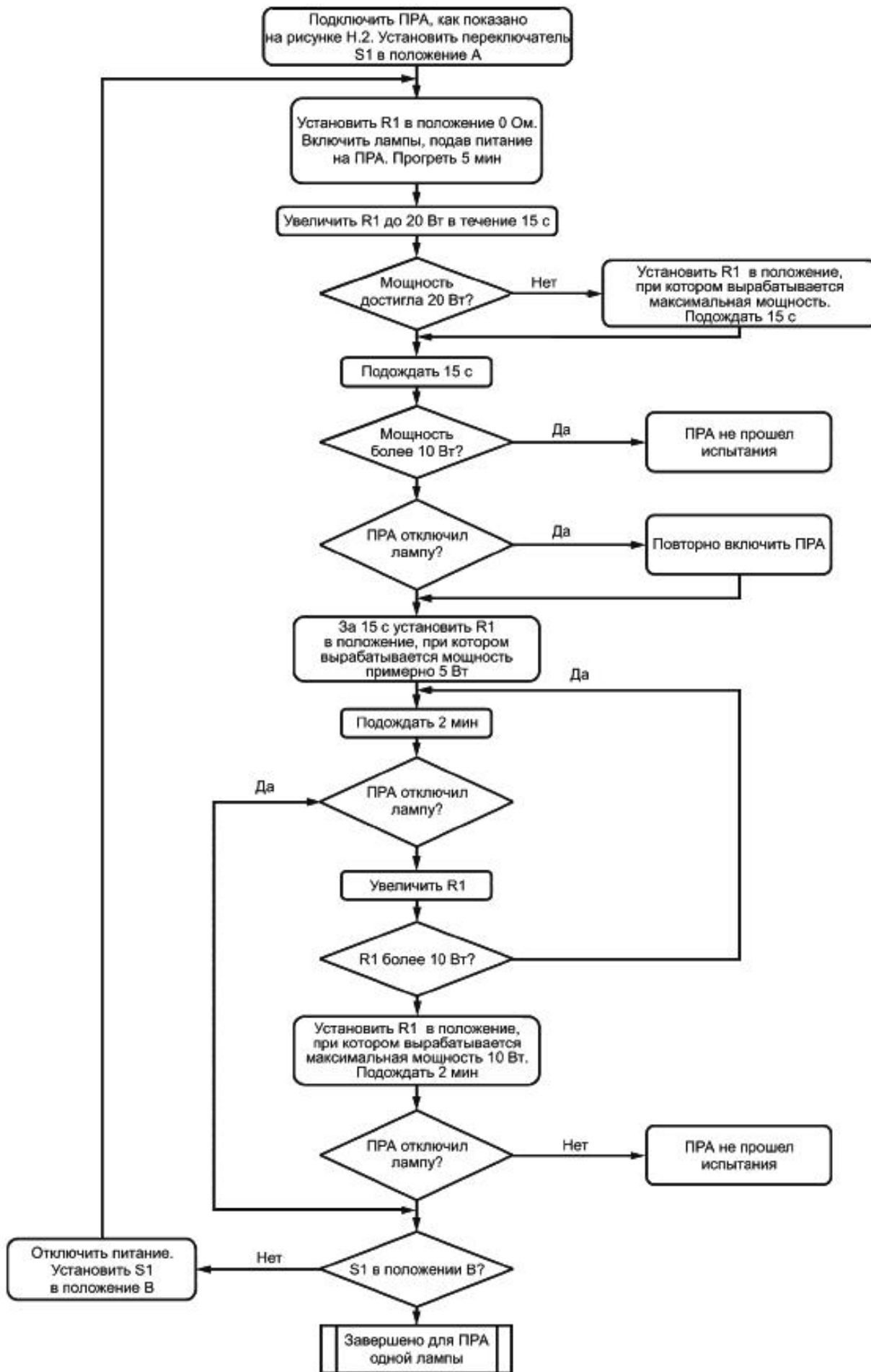
Рисунок Н.3 - Блок-схема испытания асимметричной мощностью
