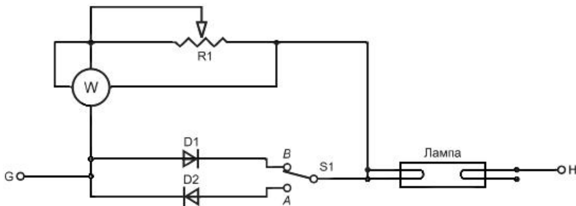
Рисунок Н.2 - Схема испытания асимметричной мощностью
