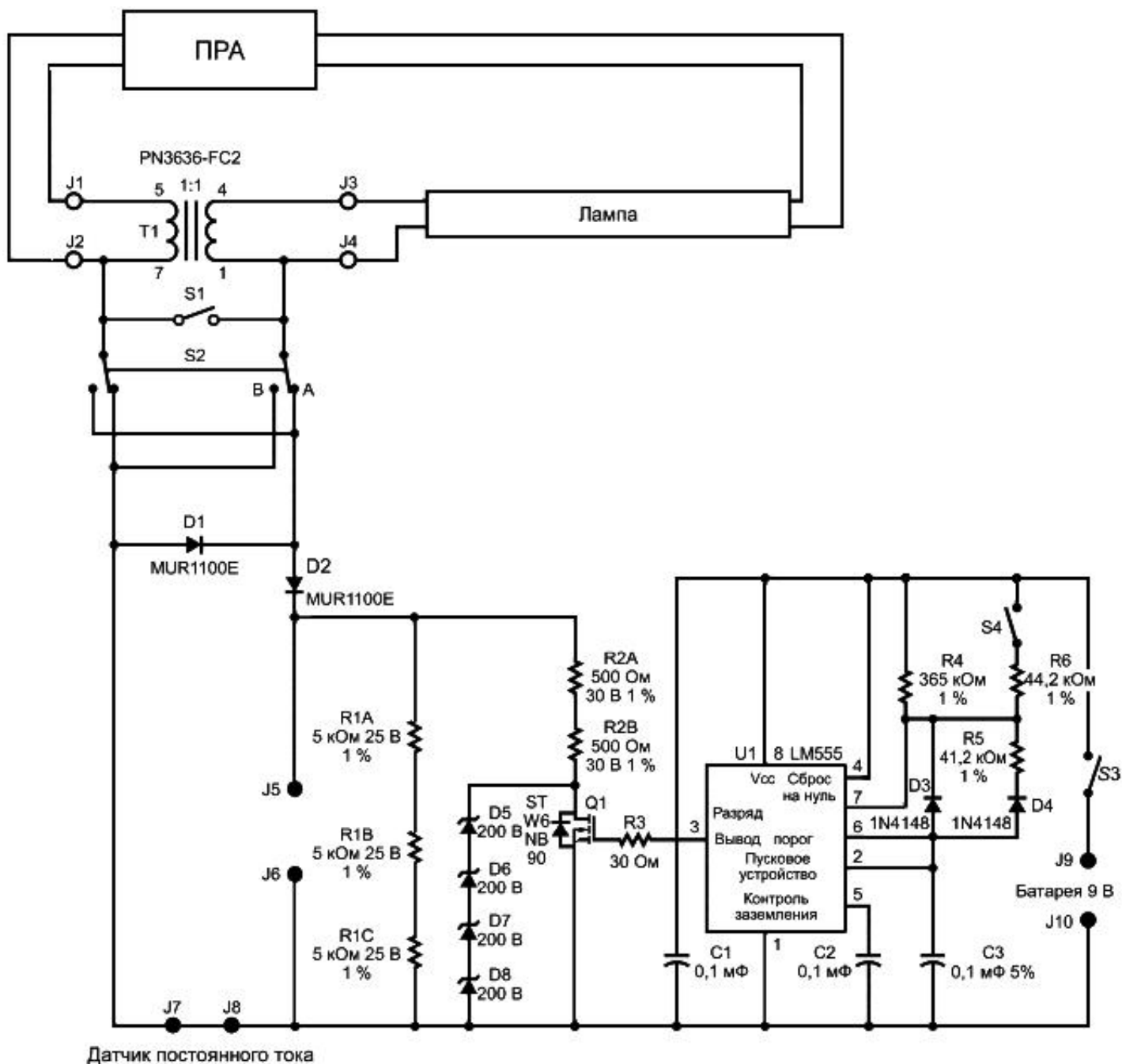
Рисунок Н.1 - Схема испытания асимметричным импульсом
